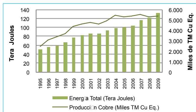
Figura 9. Evolución del consumo de energía y producción de cobre durante el periodo 1995-2009
