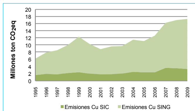
Figura 10. Evolución de emisiones de CO 2 de la minería del cobre de Chile según matriz energética durante el periodo 1995-2009
