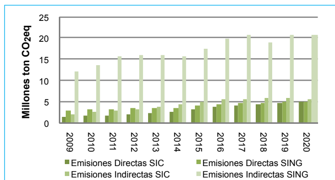
Figura 11. Proyección de emisiones directas e indirectas de GEI del sector de la minería del cobre en Chile, por sistema eléctrico Fuente: Comisión Chilena del Cobre, COCHILCO (2009)
