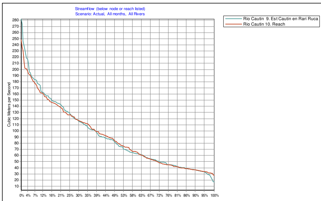
Figura 2.1-3: Curva de duración cuenca Cautín en Rari-Ruca
