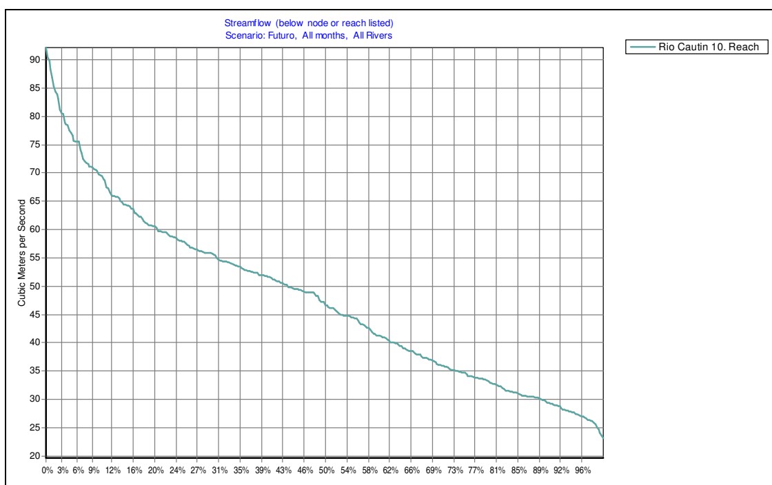
Figura 4.1-3: Curva de duración para la cuenca Cautín en Rari-Ruca (datos futuros)
