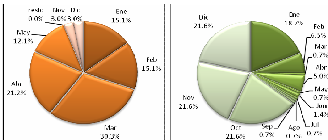
Figura 5.1-4: Probabilidad de ocurrencia del estrés hídrico actual (izquierda) y futura (derecha) del 85% de demanda a nivel mensual para la cuenca río Cautín en Rari-Ruca.
