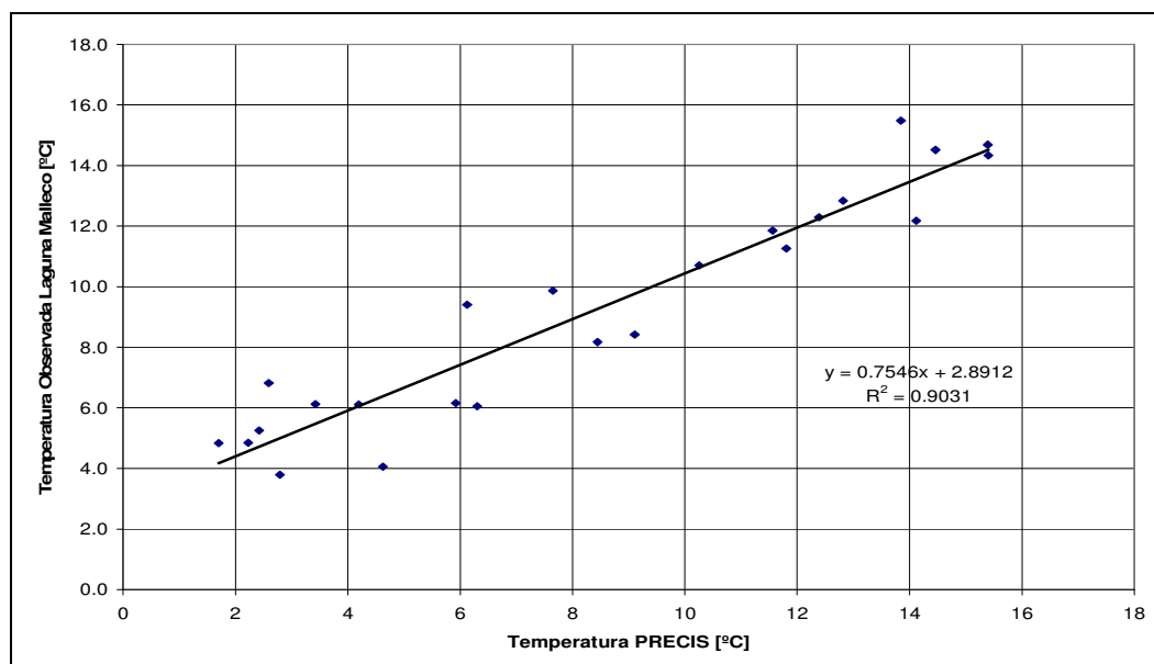
Figura 3.1-3: Corrección de temperatura simulada PRECIS. Cuenca Cautín en Rari-Ruca
