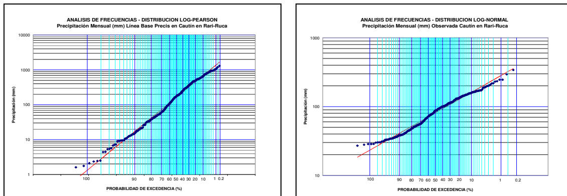
Figura 3.1-1: Análisis de frecuencia de precipitación línea base, modelo PRECIS (izquierda) y precipitación observada (derecha). Cuenca Cautín en Rari-Ruca
