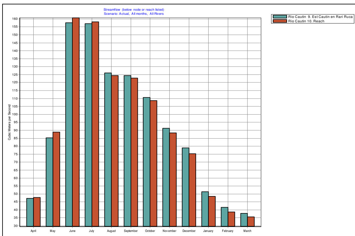
Figura 2.1-1: Calibración promedio mensual cuenca Cautín en Rari-Ruca
