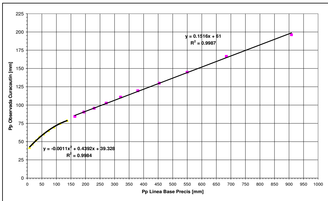
Figura 3.1-2: Corrección de precipitación simulada PRECIS. Cuenca Cautín en Rari-Ruca
