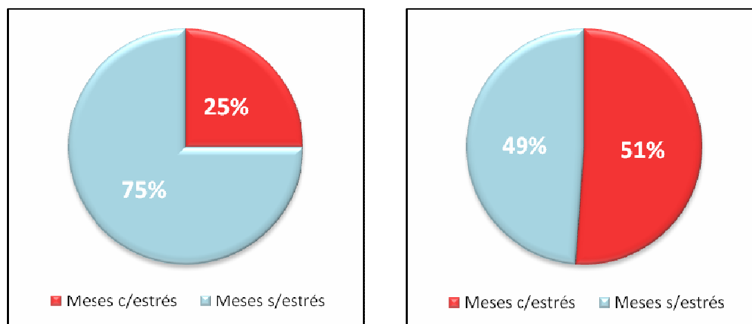
Figura 5.1-1: Estrés hídrico actual (izquierda) y futuro (derecha) para la cuenca río Cautín en Rari-Ruca. Demanda 75%
