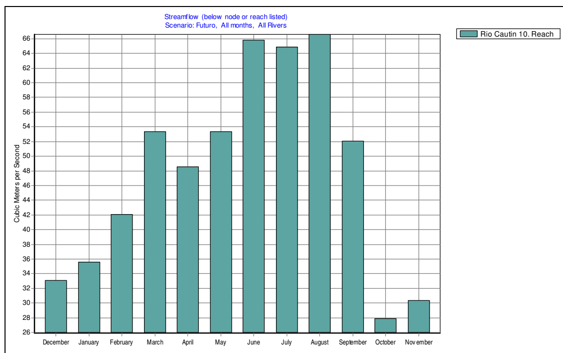
Figura 4.1-1: Promedio mensual para la cuenca Cautín en Rari-Ruca (datos futuros)
