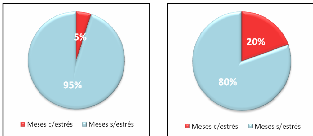
Figura 5.1-5: Estrés hídrico actual (izquierda) y futuro (derecha) para la cuenca río Cautín en Rari-Ruca. Demanda 95%
