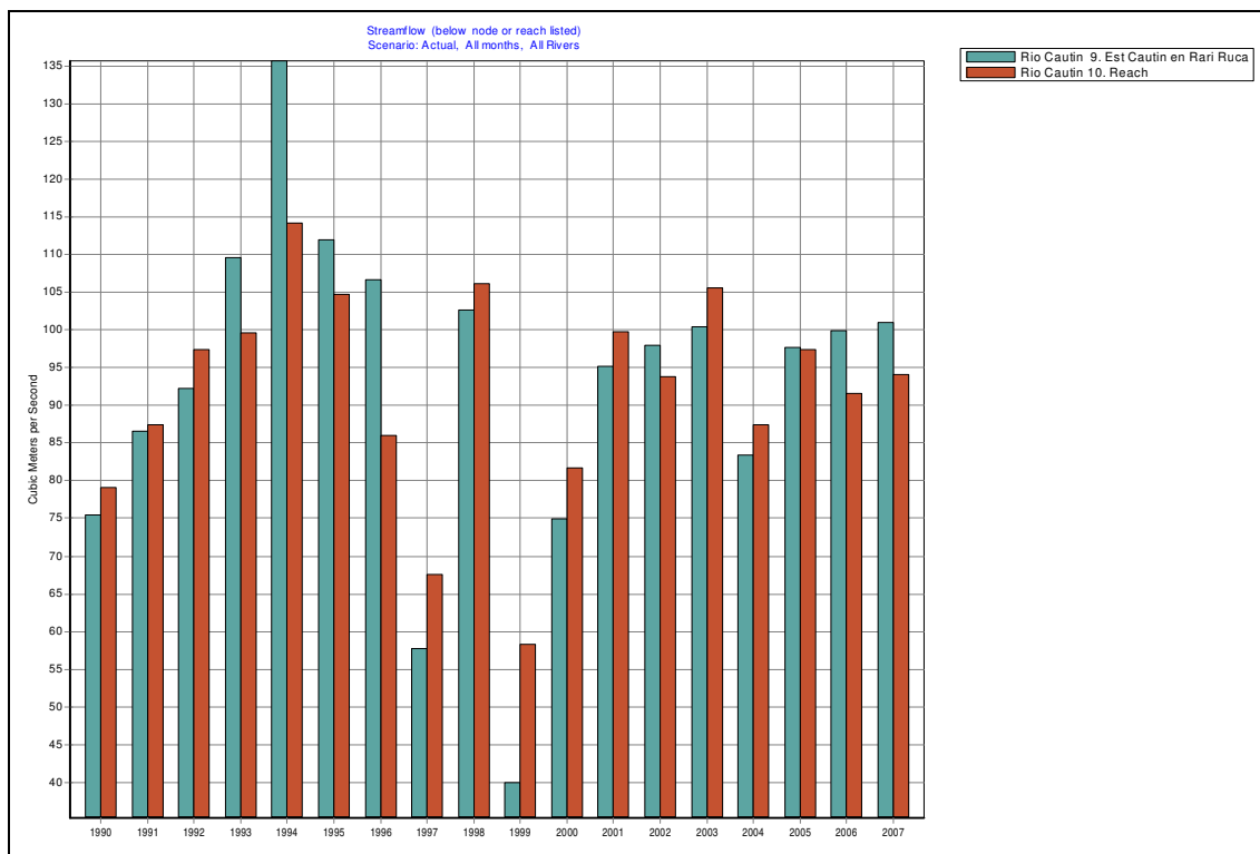
Figura 2.1-2: Calibración total anual cuenca Cautín en Rari-Ruca
