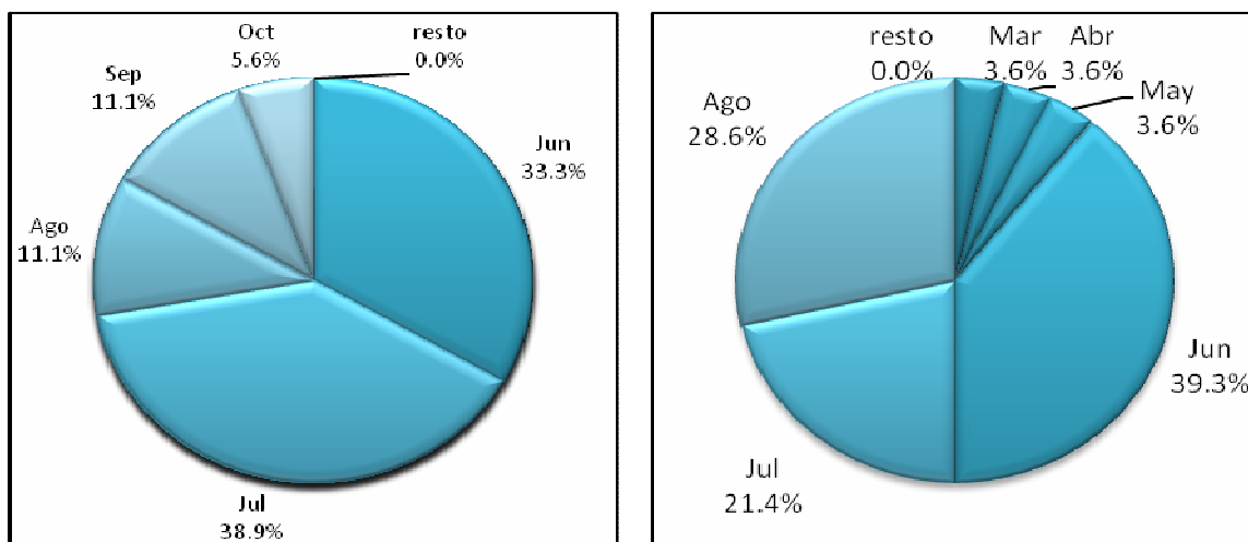
Figura 5.1-8: Caudales máximos actuales (izquierda) y futuros (derecha) para la cuenca río Cautín en Rari-Ruca
