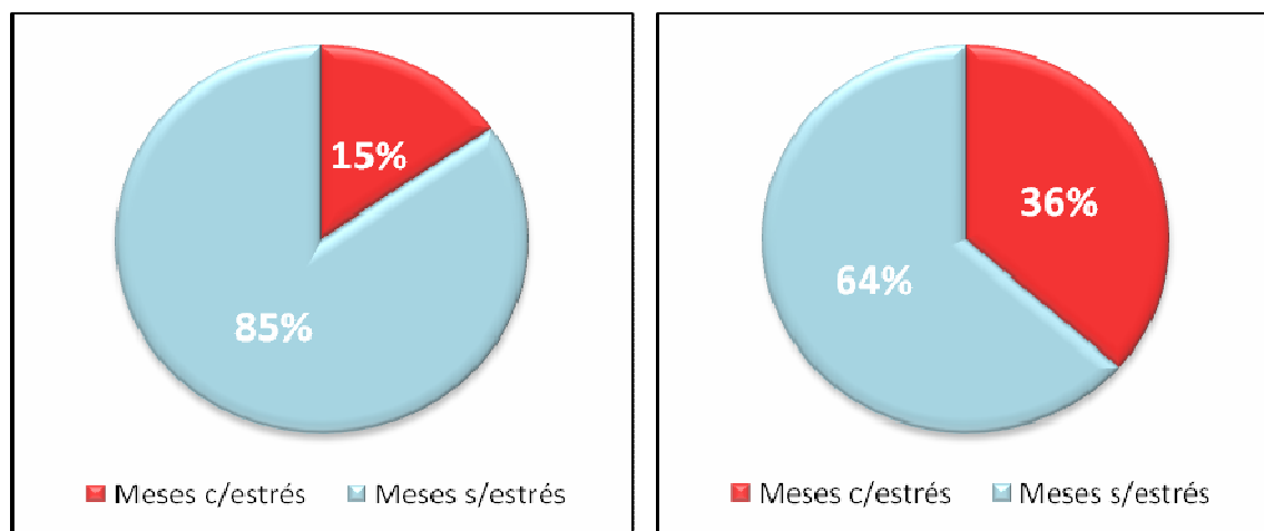
Figura 5.1-3: Estrés hídrico actual (izquierda) y futuro (derecha) para la cuenca río Cautín en Rari-Ruca. Demanda 85%
