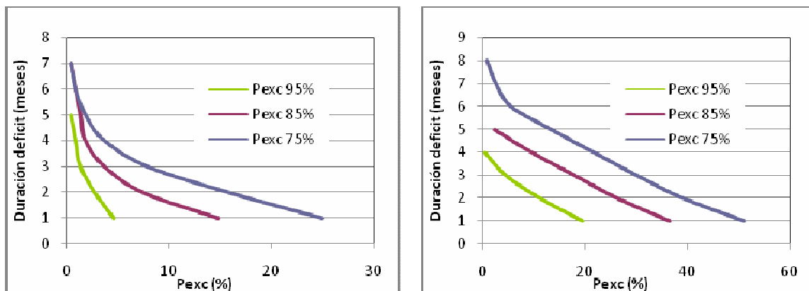
Figura 5.1-7: Curva de Duración de la duración del déficit actual (izquierda) y futuro (derecha) para la cuenca río Cautín en Rari-Ruca
