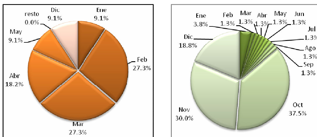
Figura 5.1-6: Probabilidad de ocurrencia del estrés hídrico actual (izquierda) y futura (derecha) del 95% de demanda a nivel mensual para la cuenca río Cautín en Rari-Ruca.
