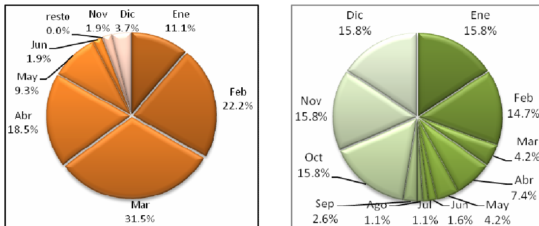
Figura 5.1-2: Probabilidad de ocurrencia del estrés hídrico actual (izquierda) y futura (derecha) del 75% de demanda a nivel mensual para la cuenca río Cautín en Rari-Ruca
