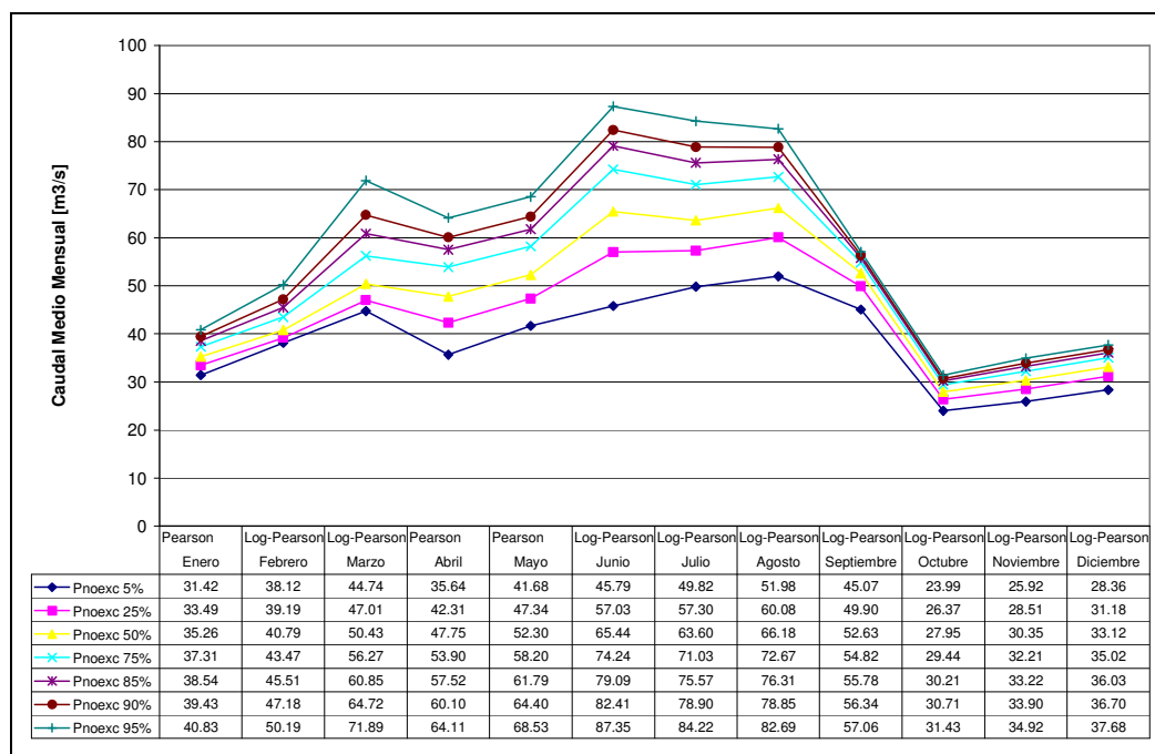
Figura 5.1-9: Curva de variación estacional (futuro) para la cuenca Cautín en Rari-Ruca
