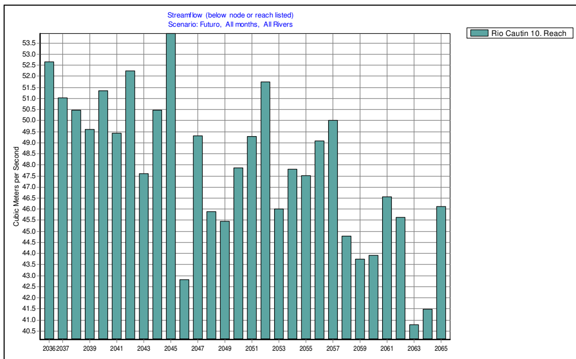
Figura 4.1-2: Total anual para la cuenca Cautín en Rari-Ruca (datos futuros)
