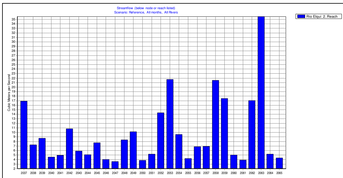
Figura 4.1-2: Total anual para la cuenca río Elqui en Algarrobal (datos futuros)
