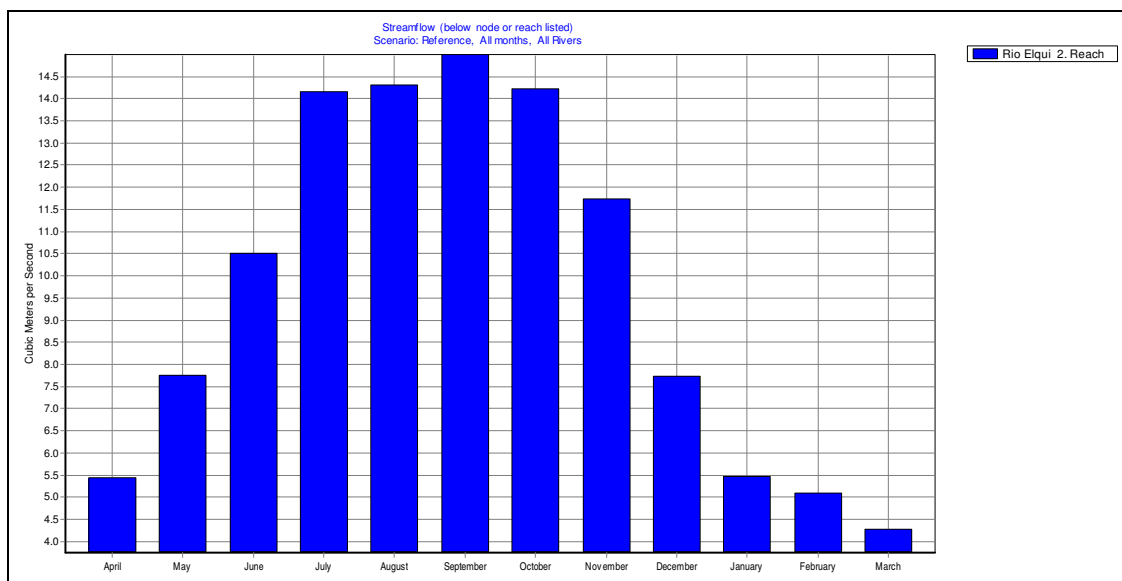
Figura 4.1-1: Promedio mensual para la cuenca río Elqui en Algarrobal (datos futuros)
