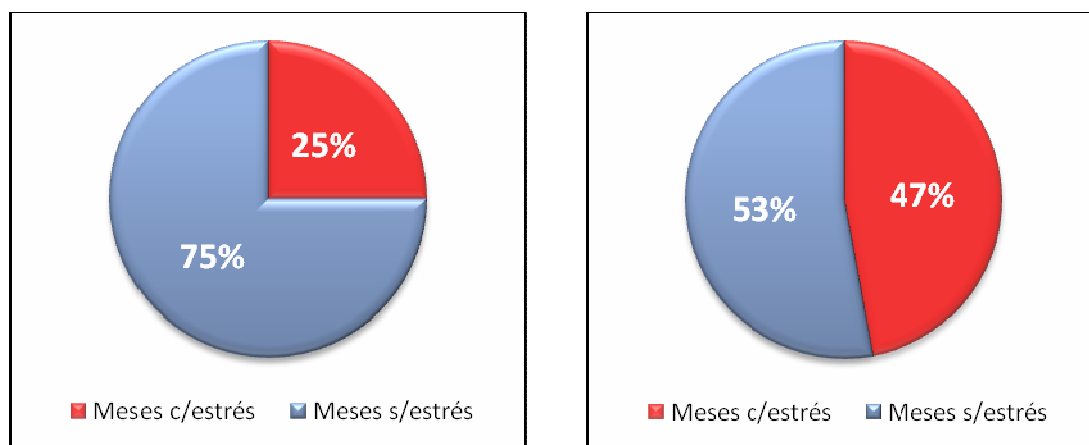
Figura 5.1-1: Estrés hídrico actual (izquierda) y futuro (derecha) para la cuenca río Elqui en Algarrobal. Demanda 75%
