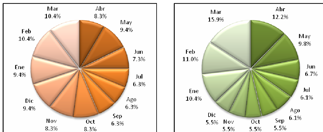
Figura 5.1-2: Probabilidad de ocurrencia del estrés hídrico actual (izquierda) y futuro (derecha) del 75% de demanda a nivel mensual para la cuenca río Elqui en Algarrobal
