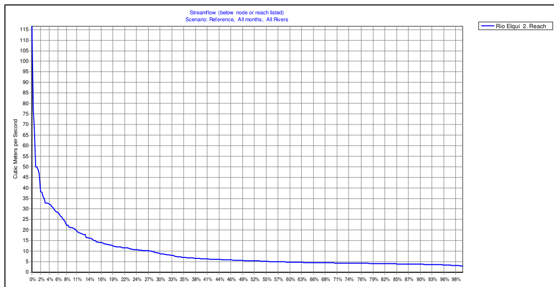
Figura 4.1-3: Curva de duración para la cuenca río Elqui en Algarrobal (datos futuros)
