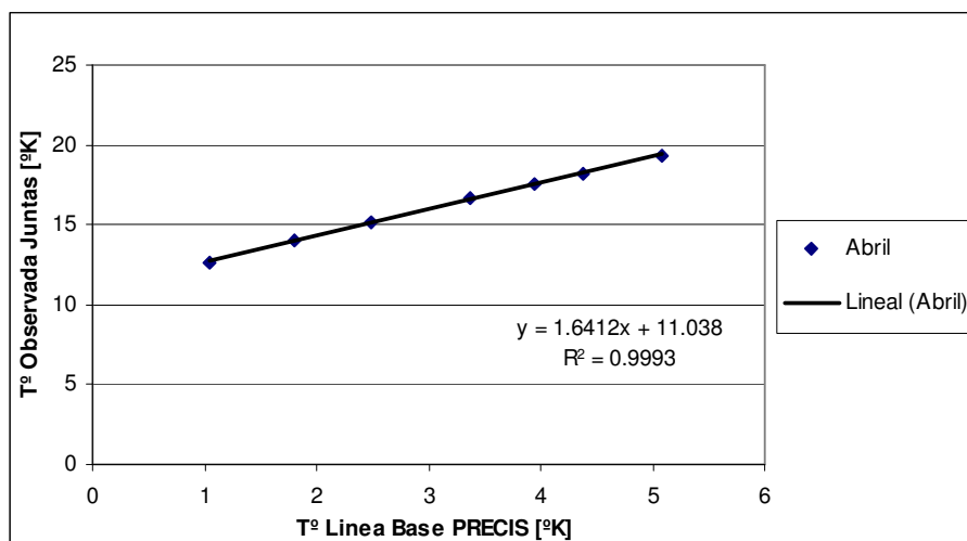
Figura 3.1-4: Corrección de temperatura simulada PRECIS en mes de abril. Cuenca río Elqui en Algarrobal
