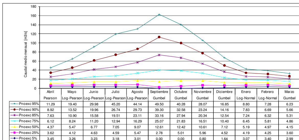
Figura 5.1-9: Curva de variación estacional (futuro) para la cuenca río Elqui en Algarrobal
