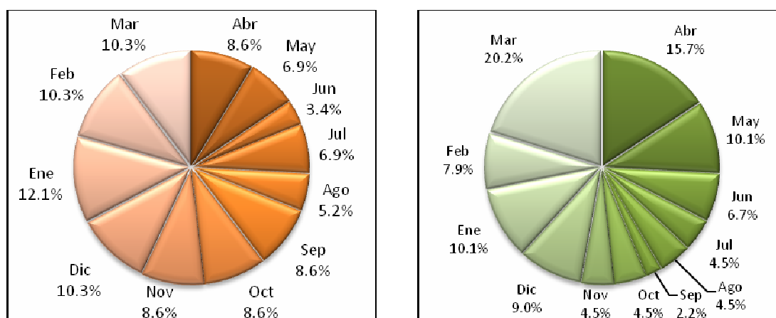
Figura 5.1-4: Probabilidad de ocurrencia del estrés hídrico actual (izquierda) y futuro (derecha) del 85% de demanda a nivel mensual para la cuenca río Elqui en Algarrobal
