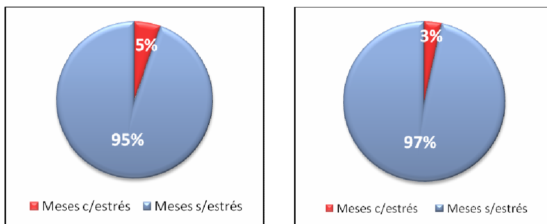
Figura 5.1-5: Estrés hídrico actual (izquierda) y futuro (derecha) para la cuenca río Elqui en Algarrobal. Demanda 95%
