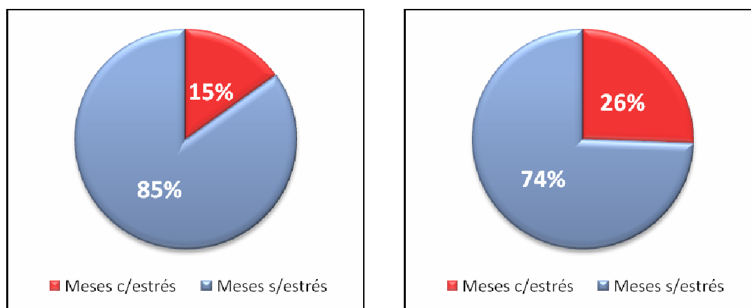
Figura 5.1-3: Estrés hídrico actual (izquierda) y futuro (derecha) para la cuenca río Elqui en Algarrobal. Demanda 85%
