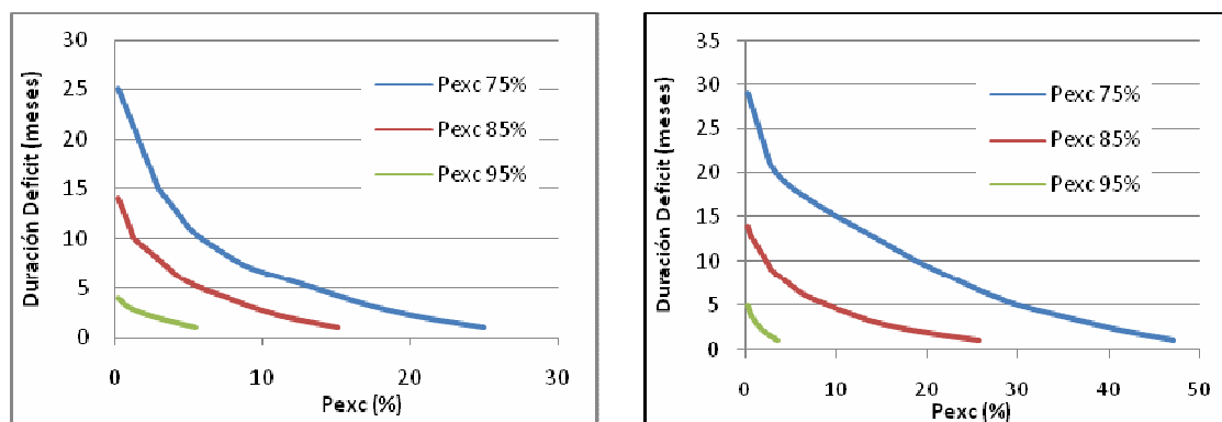
Figura 5.1-7: Curva de Duración de la duración del déficit actual (izquierdo) y futuro (derecho) para la cuenca río Elqui en Algarrobal
