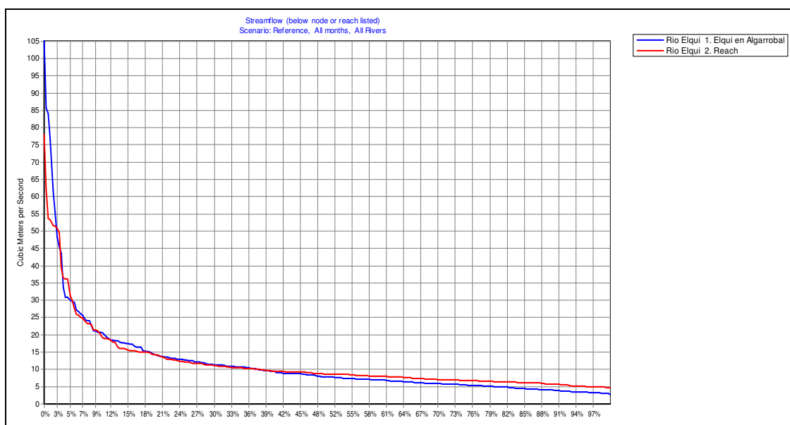
Figura 2.1-3: Curva de duración cuenca río Elqui en Algarrobal
