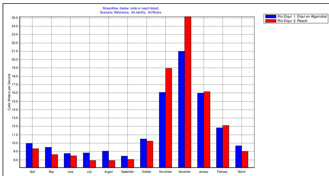
Figura 2.1-1: Calibración promedio mensual cuenca río Elqui en Algarrobal
