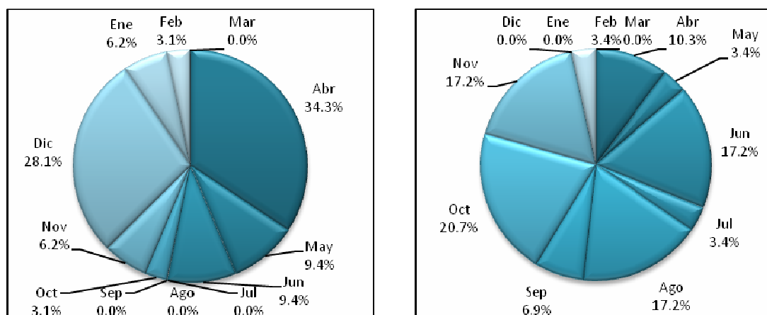
Figura 5.1-8: Caudales máximos actuales (izquierda) y futuros (derecha) para la cuenca río Elqui en Algarrobal
