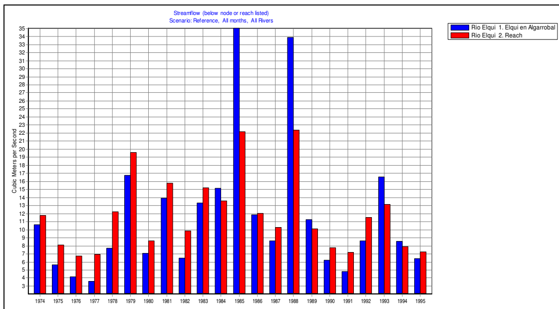
Figura 2.1-2: Calibración total anual cuenca río Elqui en Algarrobal
