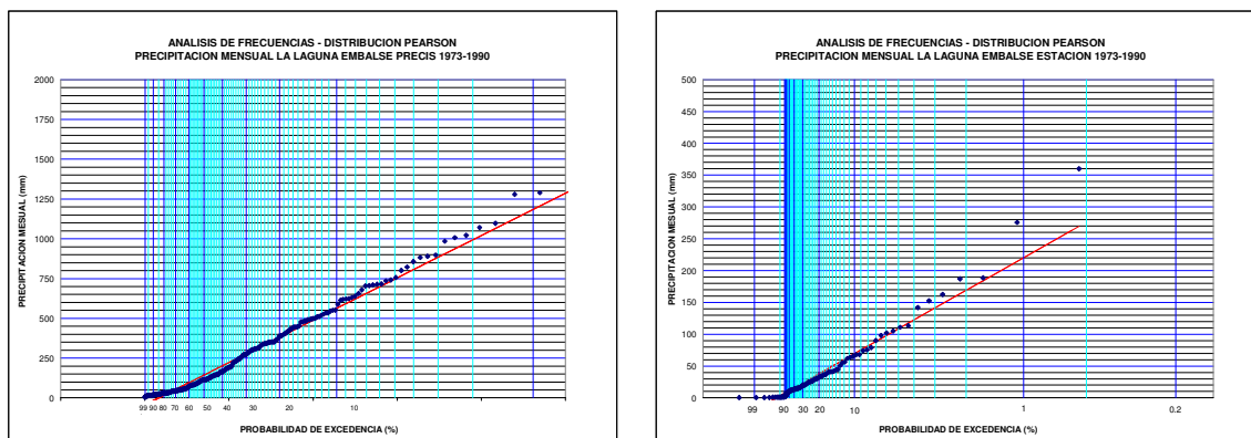
Figura 3.1-1 Análisis de frecuencia de precipitación línea base, modelo PRECIS (izquierda) y precipitación observada (derecha) en período concurrente. Cuenca río Elqui en Algarrobal
