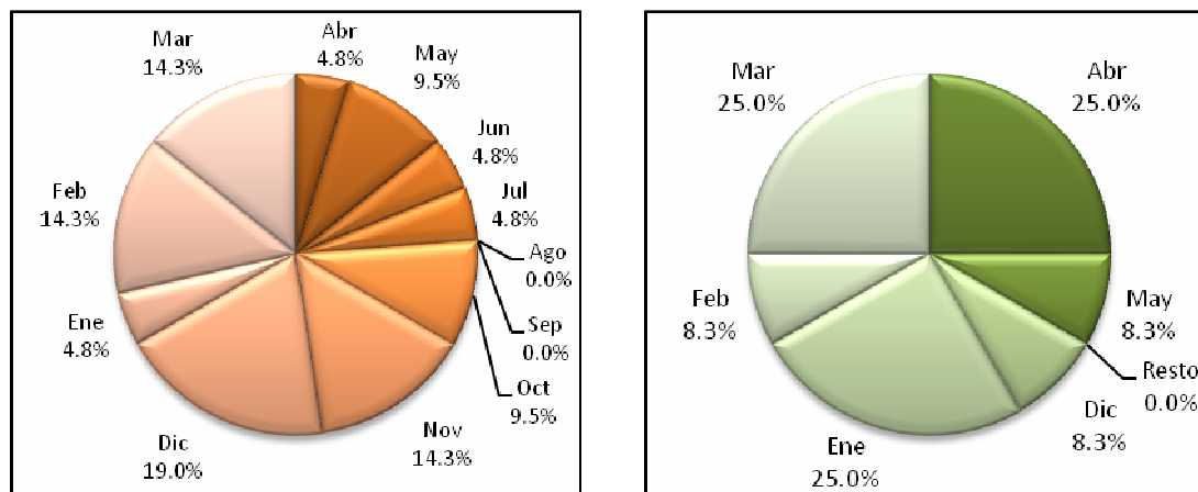
Figura 5.1-6: Probabilidad de ocurrencia del estrés hídrico actual (izq) y futuro (der) del 95% de demanda a nivel mensual para la cuenca río Elqui en Algarrobal
