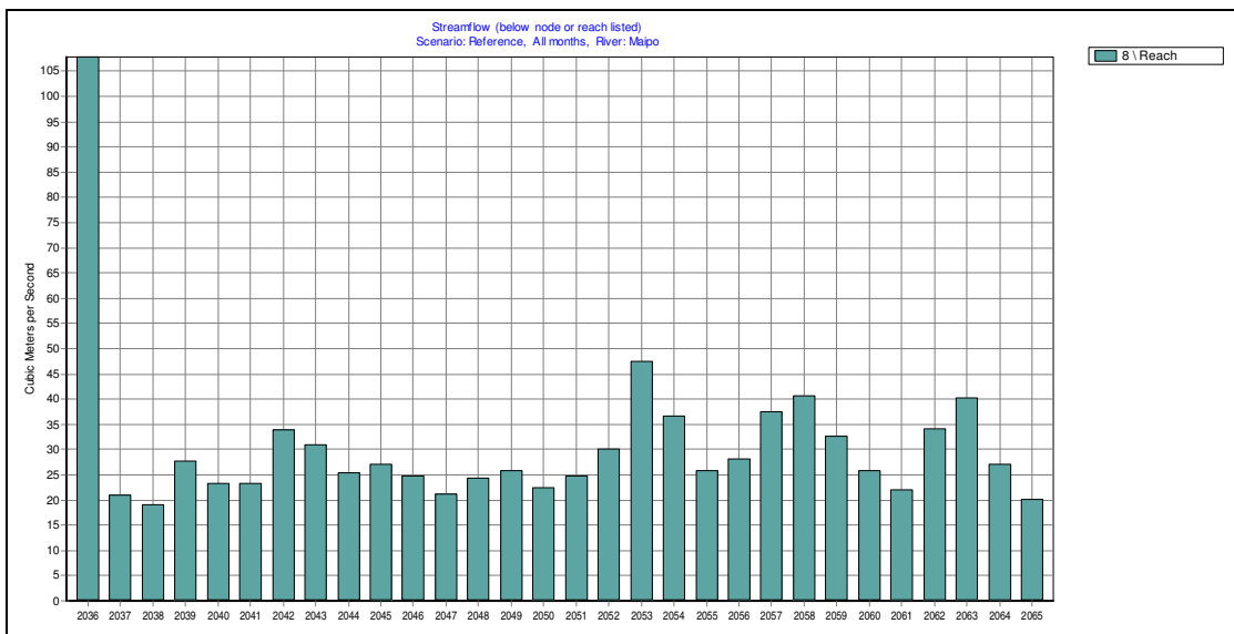
Figura 4.1-2: Total anual para la cuenca río Maipo en San Alfonso (datos futuros)
