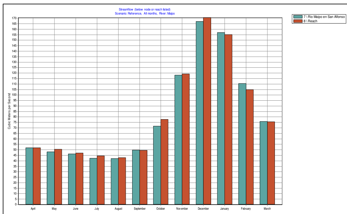
Figura 2.1-1: Calibración promedio mensual cuenca río Maipo en San Alfonso
