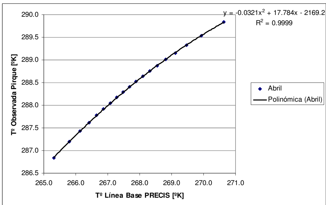
Figura 3.1-4: Corrección de temperatura simulada PRECIS en mes abril. Cuenca Maipo en San Alfonso
