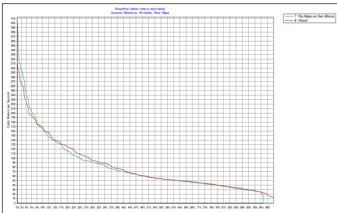
Figura 2.1-3: Curva de Duración cuenca río Maipo en San Alfonso
