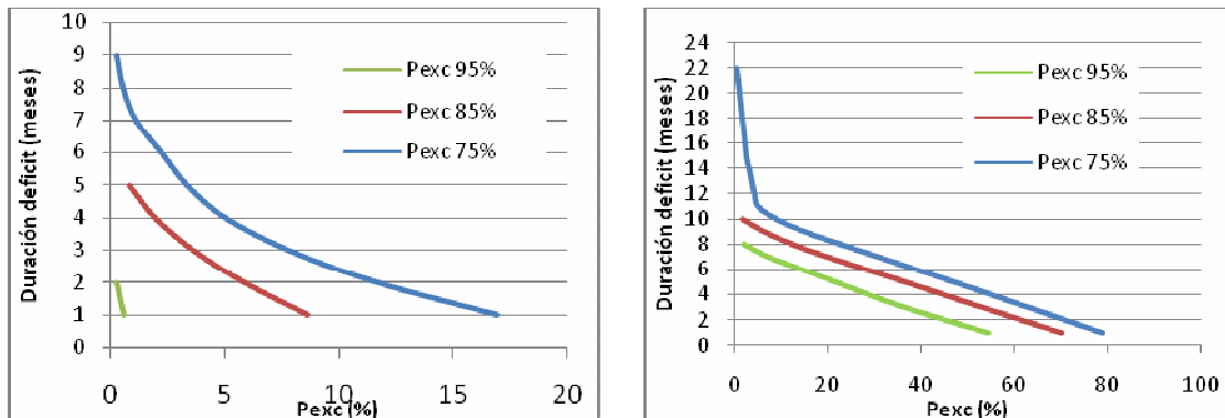
Figura 5.1-7: Curva de Duración de la duración del déficit actual (izquierda) y futuro (derecha) para la cuenca río Maipo en San Alfonso
