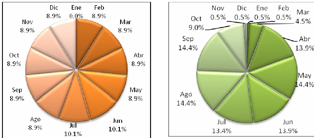
Figura 5.1-6: Probabilidad de ocurrencia del estrés hídrico actual (izquierda) y futura (derecha) del 95% de demanda a nivel mensual para la cuenca río Maipo en San Alfonso
