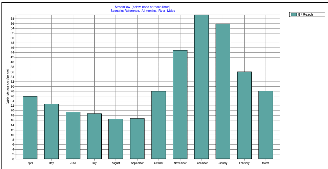
Figura 4.1-1: Promedio mensual para la cuenca río Maipo en San Alfonso (datos futuros)
