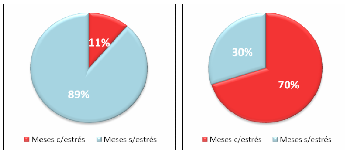
Figura 5.1-3: Estrés hídrico actual (izquierda) y futuro (derecha) para la cuenca río Maipo en San Alfonso. Demanda 85%
