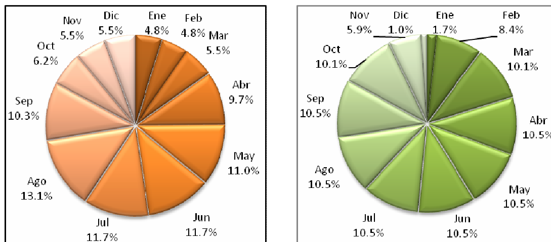
Figura 5.1-2: Probabilidad de ocurrencia del estrés hídrico actual (izquierda) y futura (derecha) del 75% de demanda a nivel mensual para la cuenca río Maipo en San Alfonso
