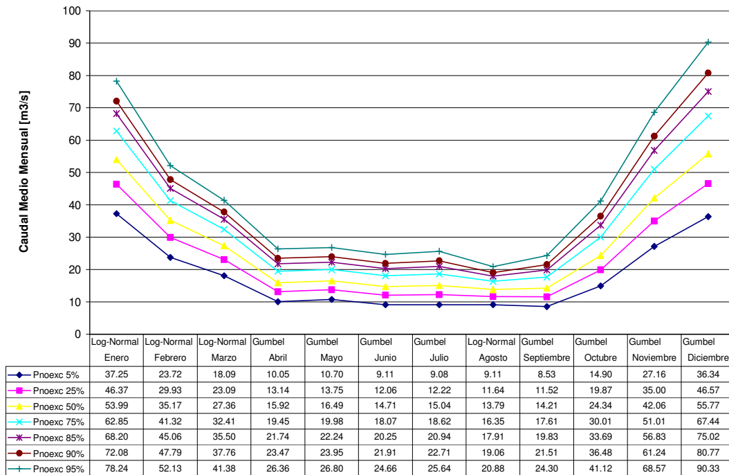
Figura 5.1-9: Curva de variación estacional (futuro) para la cuenca río Maipo en San Alfonso
