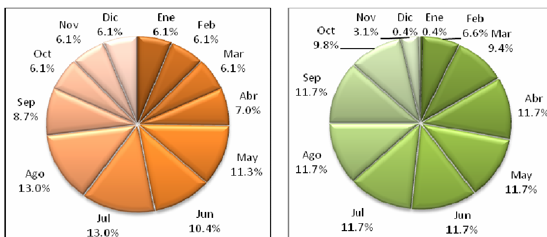
Figura 5.1-4: Probabilidad de ocurrencia del estrés hídrico actual (izquierda) y futura (derecha) del 85% de demanda a nivel mensual para la cuenca río Maipo en San Alfonso
