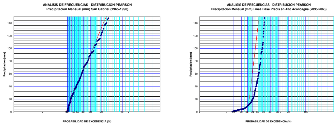
Figura 3.1-1: Análisis de frecuencia de precipitación línea base, modelo PRECIS (izquierda) y precipitación observada (derecha) en período concurrente. Cuenca Maipo en San Alfonso
