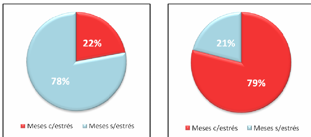
Figura 5.1-1: Estrés hídrico actual (izquierda) y futuro (derecha) para la cuenca río Maipo en San Alfonso. Demanda 75%
