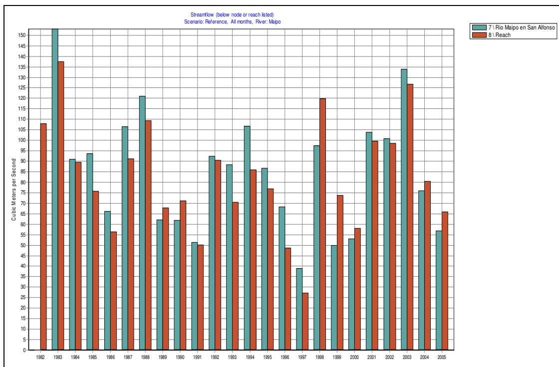
Figura 2.1-2: Calibración total anual cuenca río Maipo en San Alfonso
