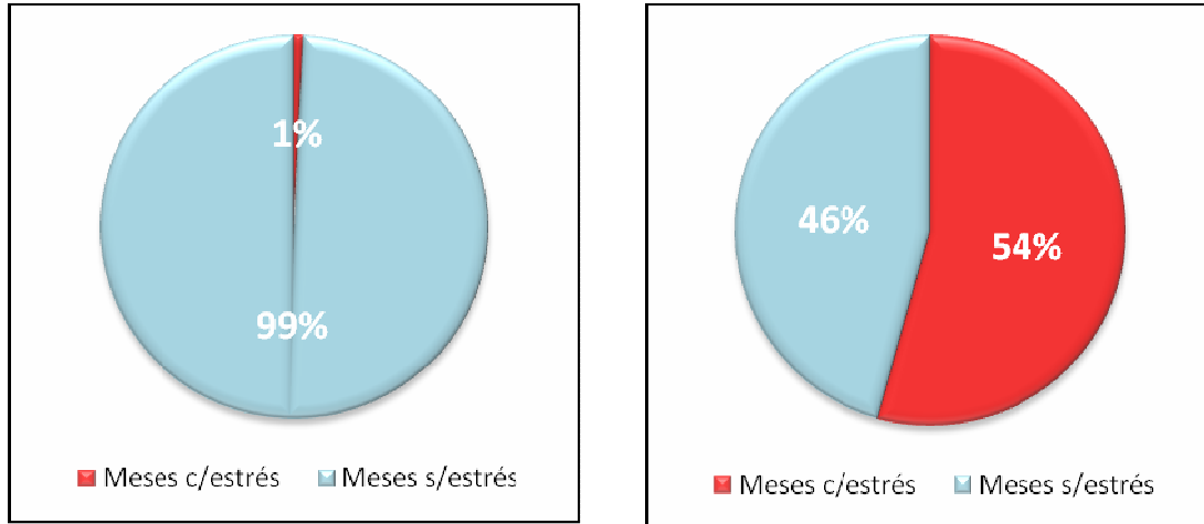
Figura 5.1-5: Estrés hídrico actual (izquierda) y futuro (derecha) para la cuenca río Maipo en San Alfonso. Demanda 95%
