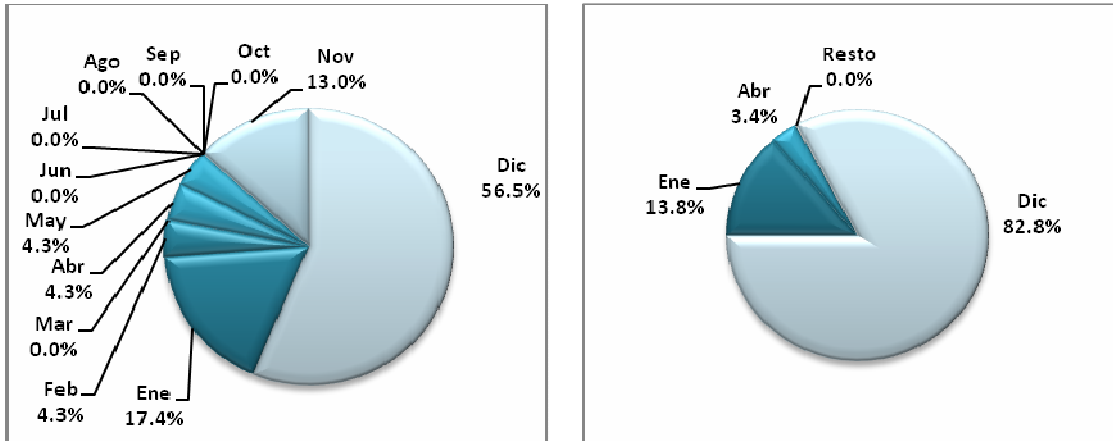
Figura 5.1-8: Caudales máximos actuales (izquierda) y futuros (derecha) para la cuenca río Maipo en San Alfonso
