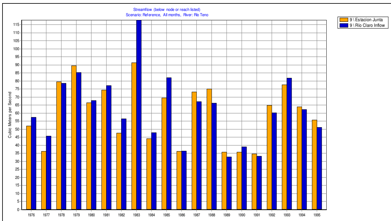
Figura 2.1-2: Calibración total anual cuenca del río Teno
