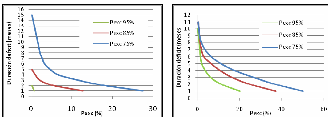
Figura 5.1-7: Curva de Duración de la duración del déficit actual (izquierda) y futura (derecha) para la cuenca andina del río Teno
