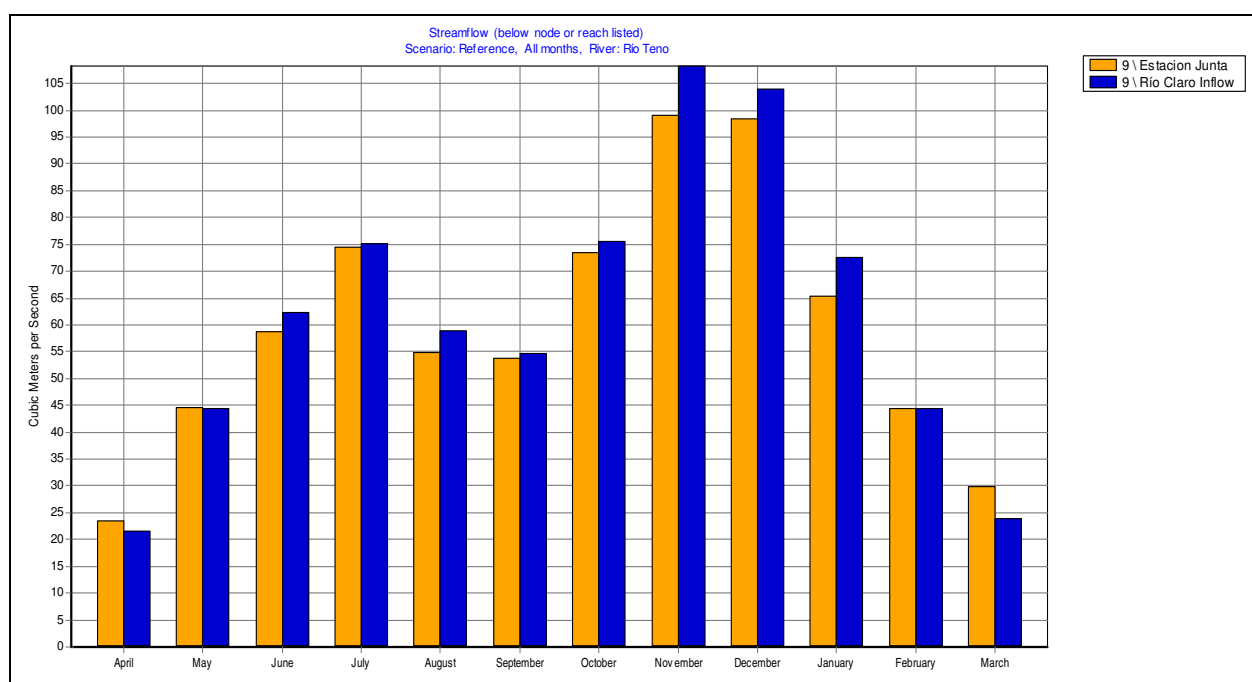
Figura 2.1-1 Calibración promedio mensual cuenca andina del río Teno
