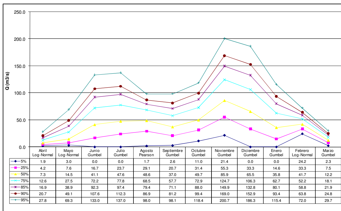
Figura 5.1-9: Curva de variación estacional (futuro) para la cuenca andina del río Teno
