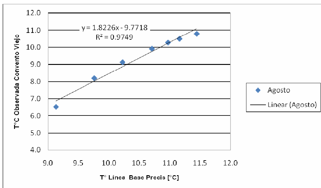
Figura 3.1-4: Corrección de precipitación simulada PRECIS en mes agosto. Cuenca andina del Tenó
