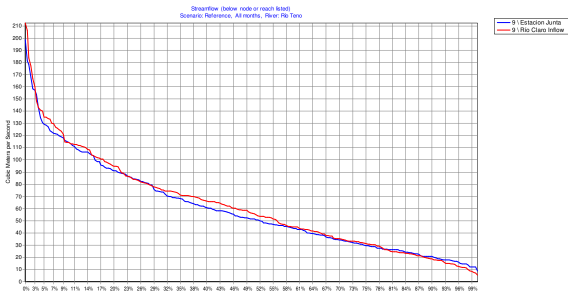
Figura 2.1-3: Curva de duración cuenca andina del río Teno
