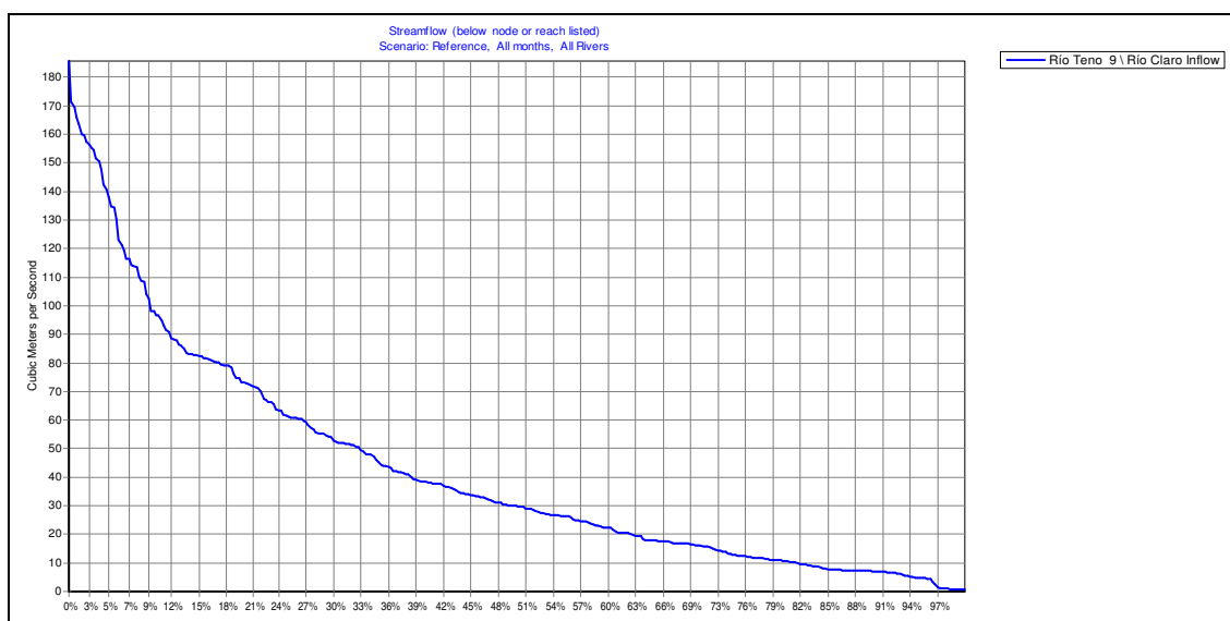
Figura 4.1-2: Curva de duración para la cuenca del río Teno (datos futuros)
