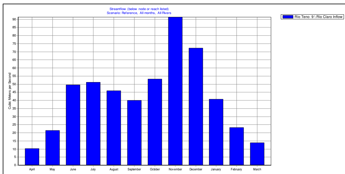
Figura 4.1-1: Caudales medios mensuales para la cuenca andina del río Teno (datos futuros)
