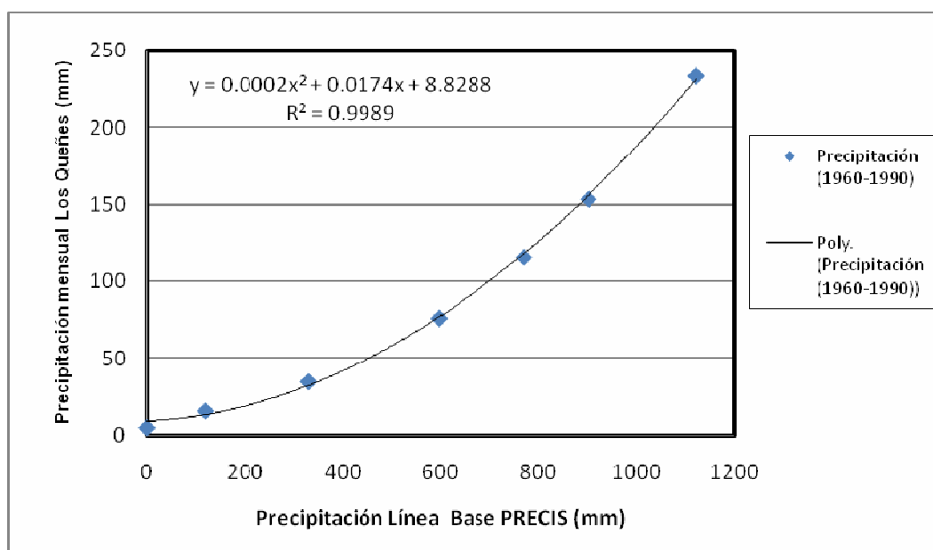
Figura 3.1-3: Corrección de precipitación simulada PRECIS en mes abril. Cuenca andina del Teno
