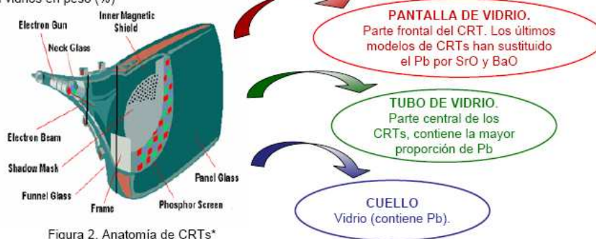
Figura 2. Anatomía de CRTs*
