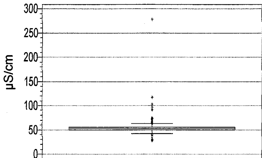
Fig. 2. Box –Plot Conductividad
