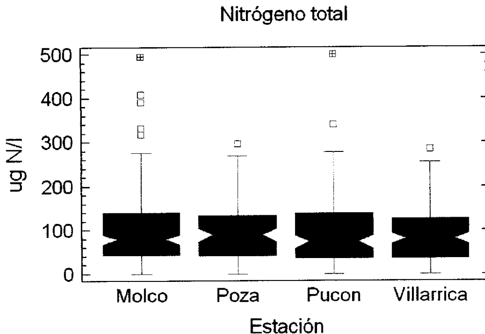
Fig.7 Nitrógeno total en las 4 estaciones de la red de monitoréo de la DGA.
