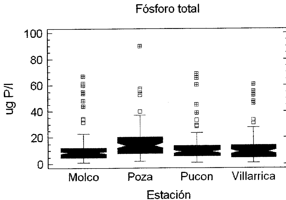
Fig.9 Fósforo total en las 4 estaciones de la red de monitoréo de la DGA.
