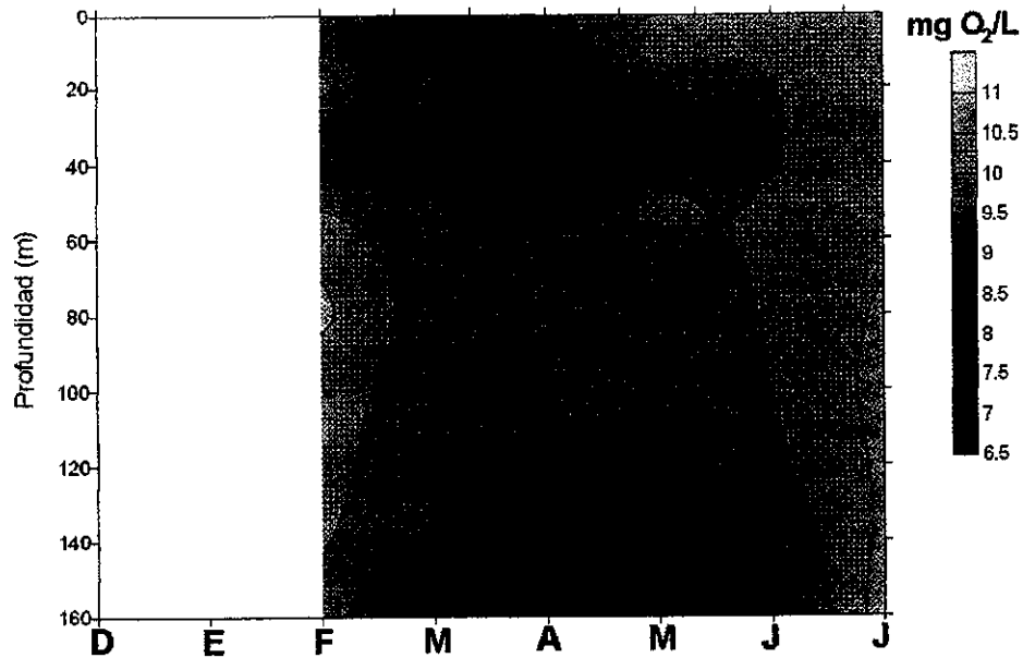
Anexo2 Fig. 3 Isopletas del oxígeno disuelto en el centro del L.Villarrica
