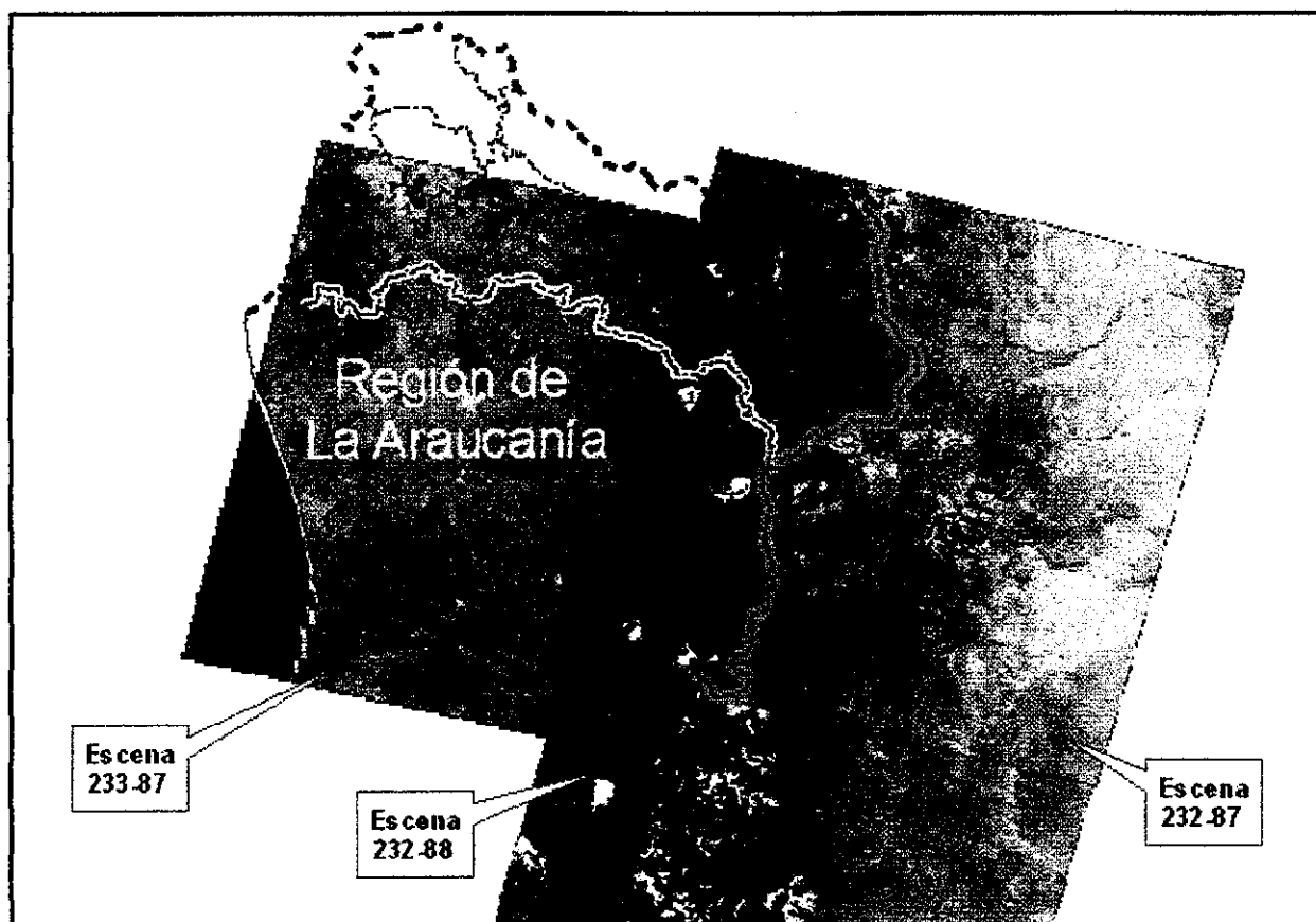
Figura 1. Mapa de ubicación de la zona de estudio y escenas adquiridas
