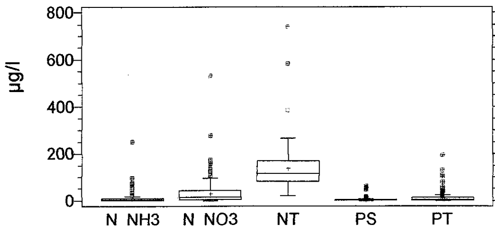
Fig.11 Amonio, nitrato, NT, P soluble y PT en el L.Villarrica (datos UACH).
