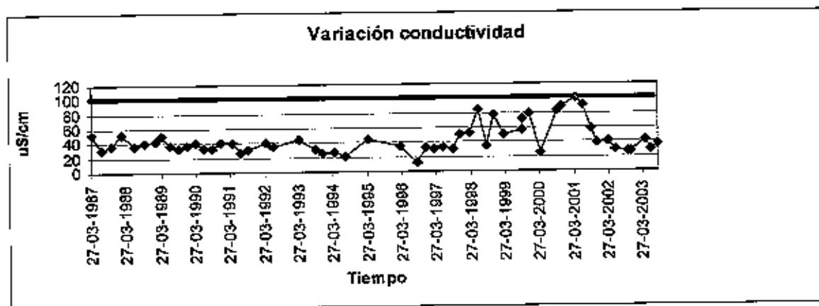
Figura 4. Variabilidad temporal en la Conductividad en el río Cruces, estación Rucaco (fuente: Minuta de CONAMA, la línea roja en el gráfico, indica el valor norma).
