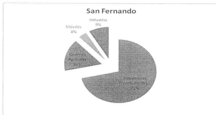
Figura 11. Emisiones de MP10 por sector para la comuna de San Fernando (Fuente: Estudio FNDR "Diagnóstico y Plan de Gestión Calidad del Aire VI Región", 2008)
