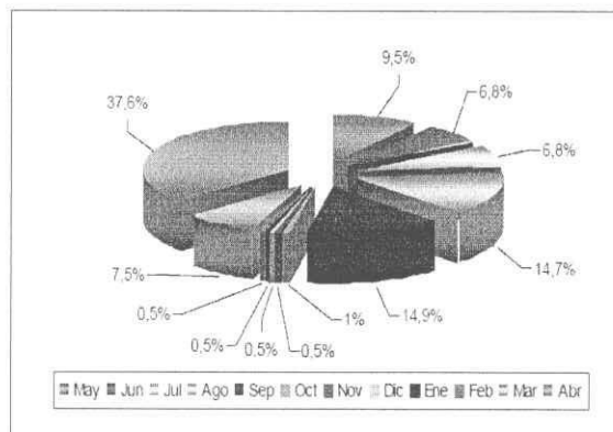
Figura 22. Distribución temporal de quemas en la zona saturada del Valle Central. (Fuente: Estudio "Medidas para el control de la contaminación por quemas, 2009")
