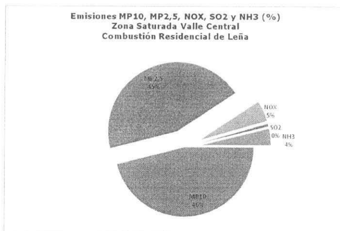
Figura 12. Emisiones de MP10, MP2,5, NO x , SO 2 y NH 3 por Combustión residencial de leña en la zona saturada del Valle Central (Fuente: Estudio FNDR "Diagnóstico y Plan de Gestión Calidad del Aire VI Región", 2008)
