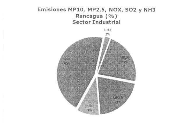
Figura 16. Emisiones de MP10, MP2,5, NO x , SO 2 y NH 3 sector industrial comuna de Rancagua (Fuente: Estudio FNDR "Diagnóstico y Plan de Gestión Calidad del Aire VI Región", 2008)
