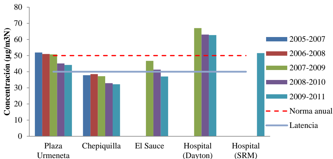
Figura 1: Concentración Trianual de MP10 ( \mu\text{g}/\text{m}^3\text{N} )
