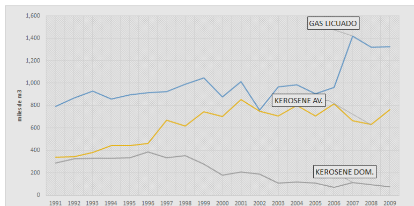
Figura 31: Producción nacional de combustibles derivado del petróleo. Fuentes: Balances Energía (hasta el 2008), ENAP (2009 y 2010).
